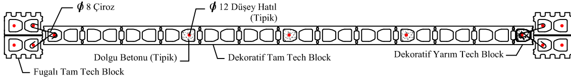
A-A KESİTİ
