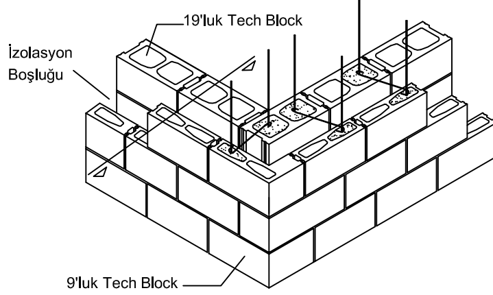
PERSPEKTİF
