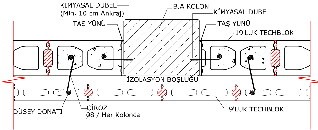
TECH BLOK GİYDİRME CEPHE DUVAR-KOLON BAĐLANTISI
