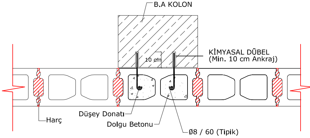
KOLON BİRLEŐİM DETAYI (TECH BLOK DIŐ YÜZEYDE)
