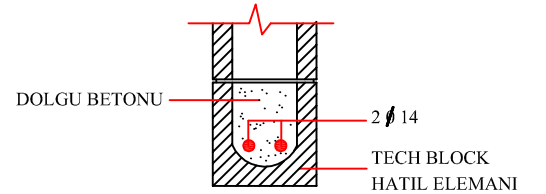
"A" DETAYI
