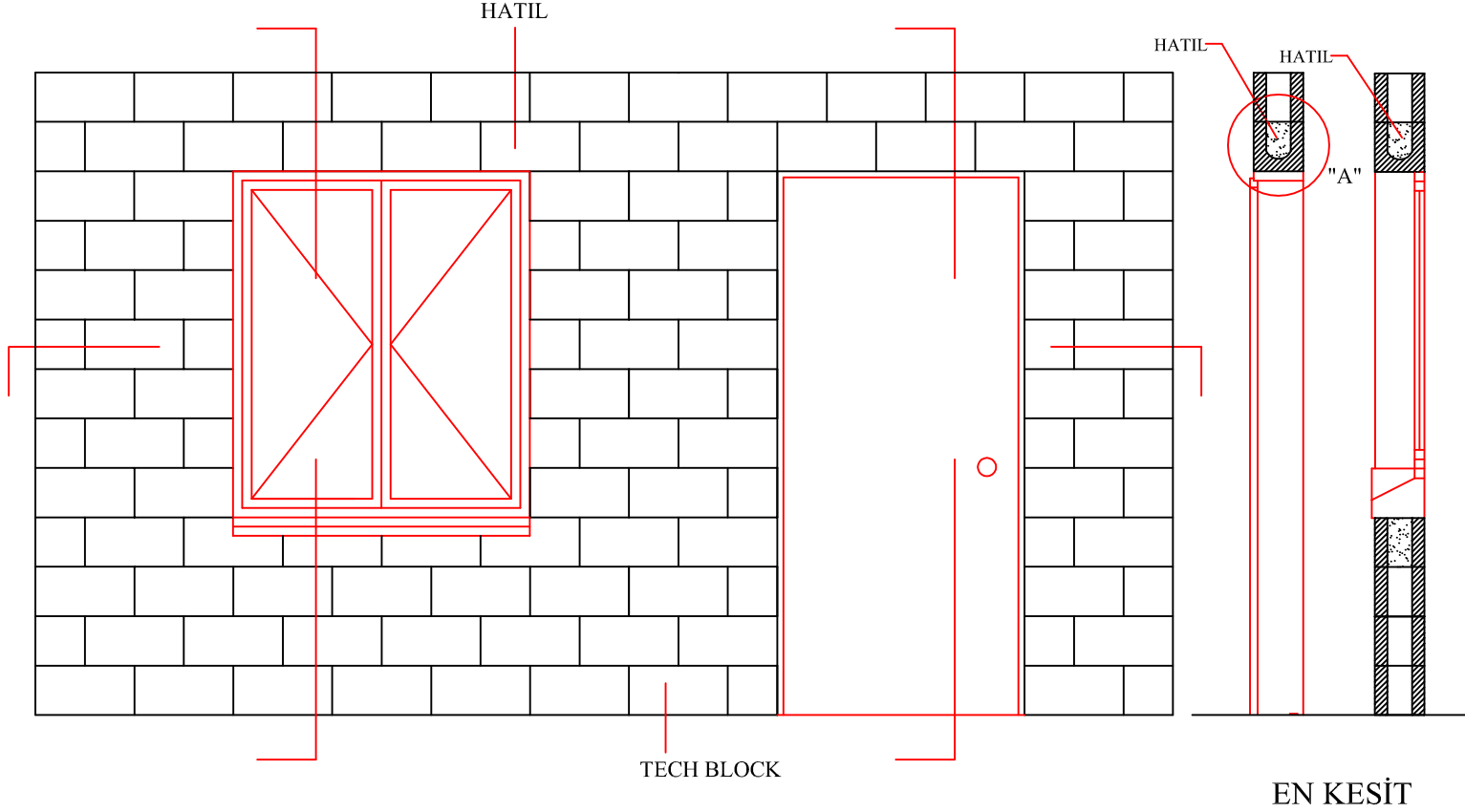
GÖRÜNÜŞ
